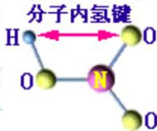
硝酸分子内的氢键
