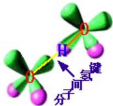
水分子间的氢键
