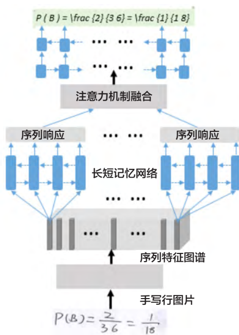
图 4: 基于深度学习的手写识别模型
