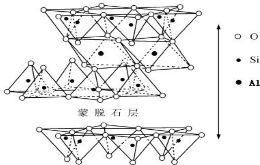
图 1 蒙脱石的层状结构图
