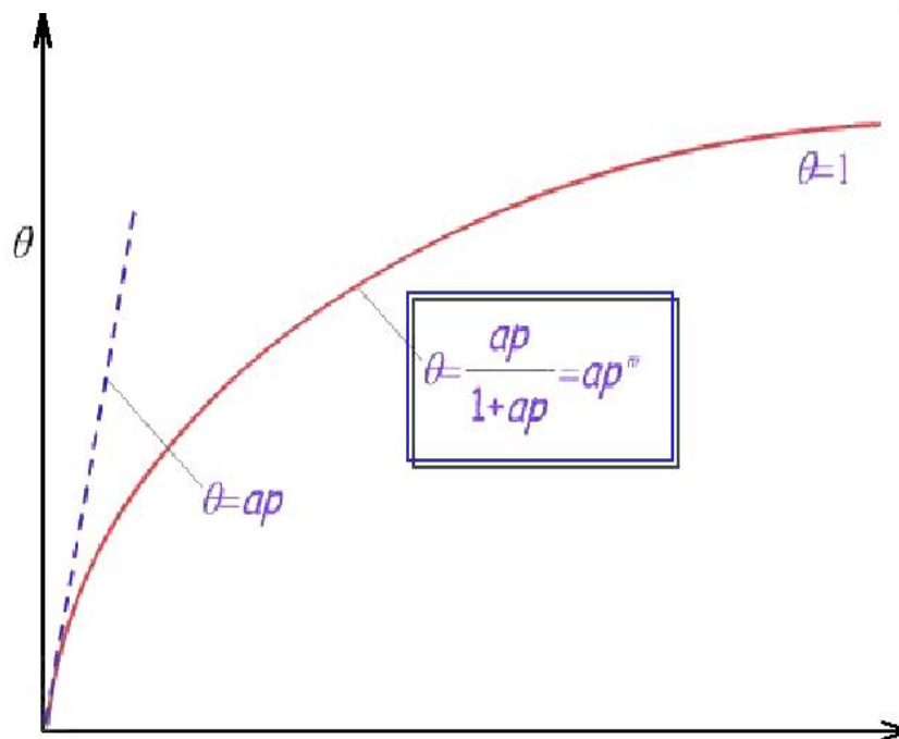
兰缪尔等温式的示意图
