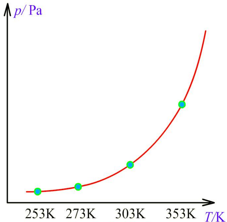
吸附等量线
