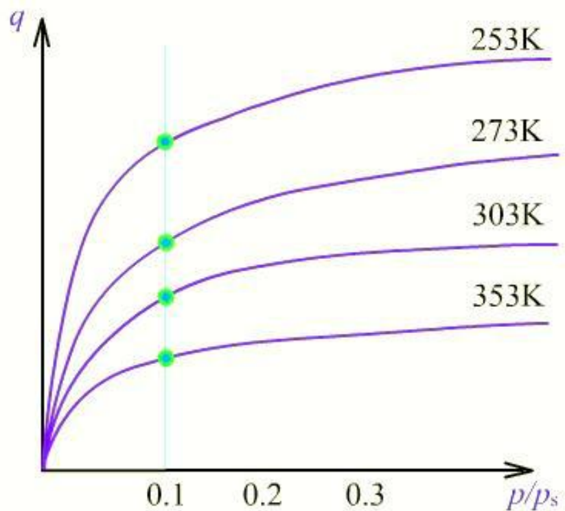
吸附等温线
