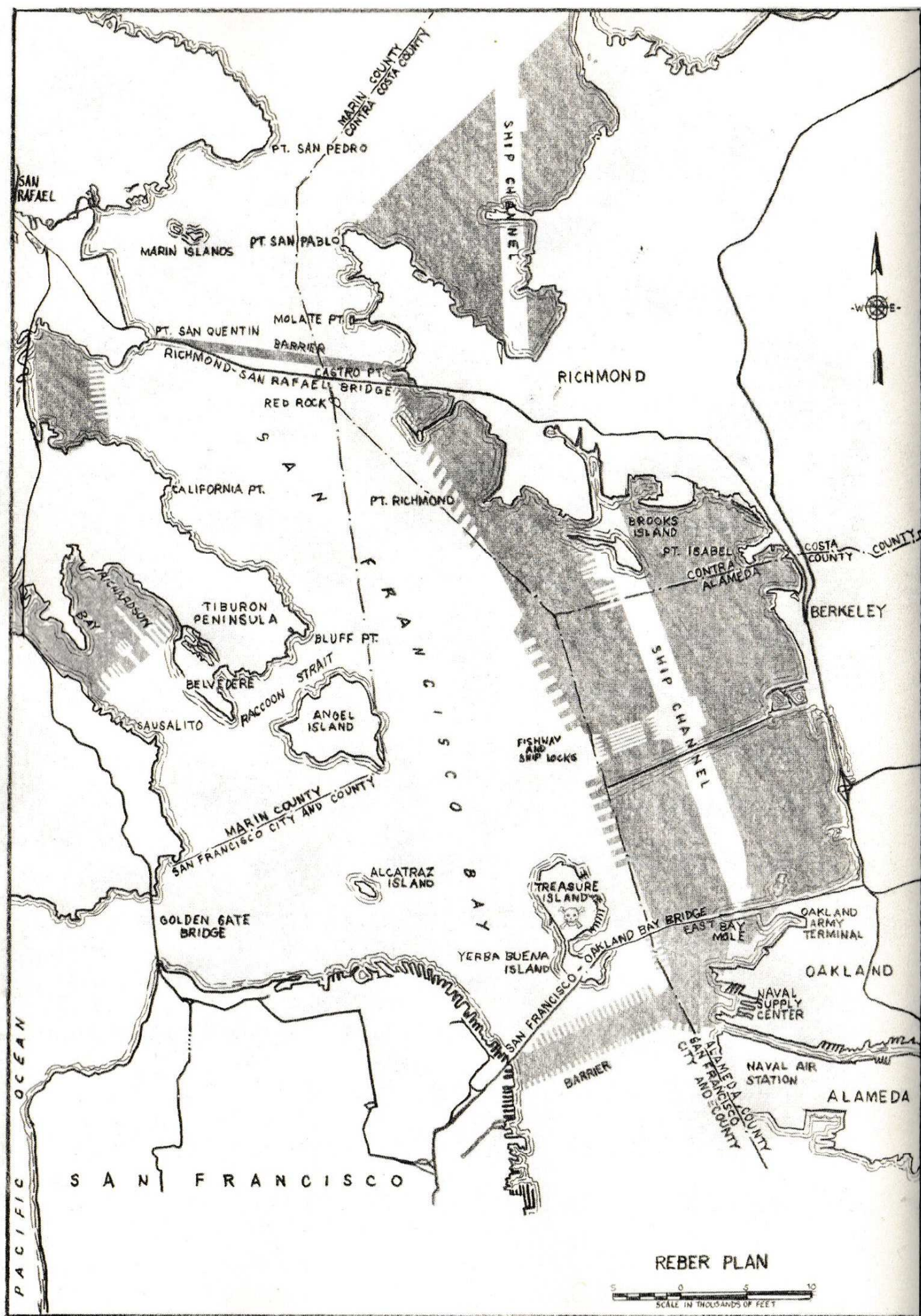
图 6-1 旧金山湾区大坝设计方案
